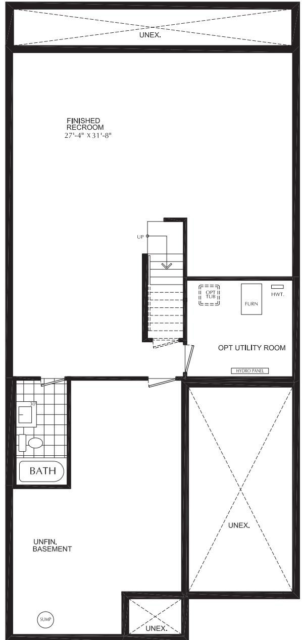
OPTIONAL BASEMENT
